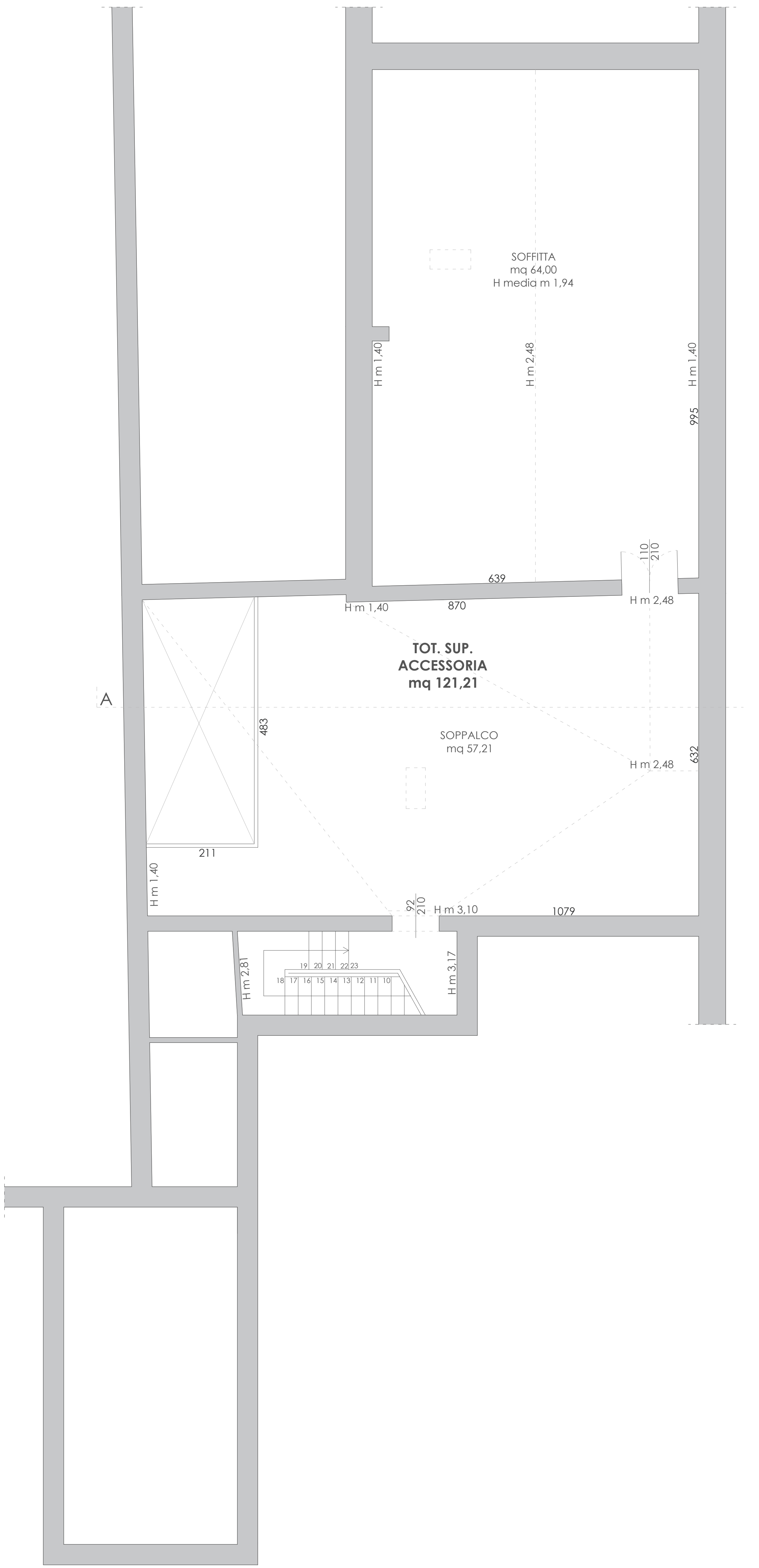
Pianta piano sottotetto S 1:50 STATO ATTUALE
