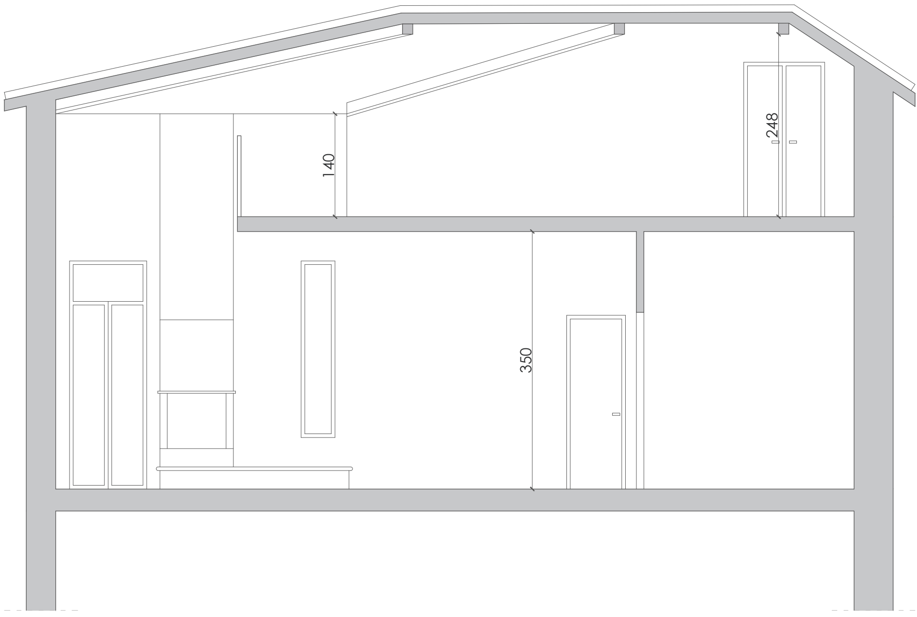
Sezione A-A' S 1:50 STATO ATTUALE
